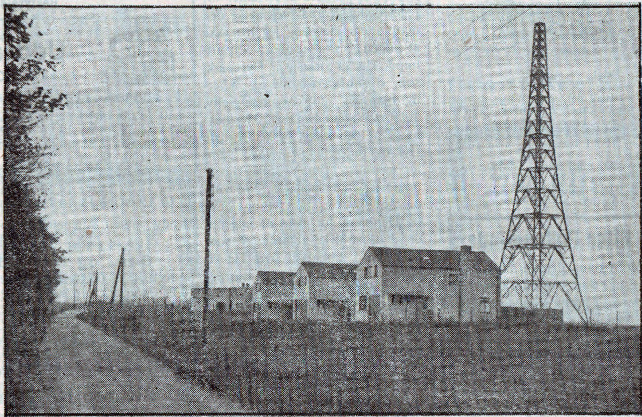
Den nye Herstedvester Radio-Senderstation.
